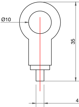
ELEVATION · OPTION C · GRIPPER RING SCALE · 1:1
