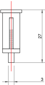
ELEVATION · OPTION B · SIDE EXIT GRIPPER SCALE · 1:1
