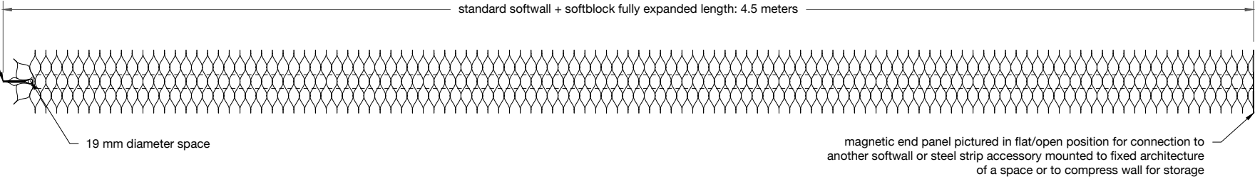
PLAN · EXPANDED
