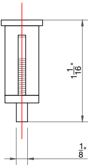
ELEVATION · OPTION B · SIDE EXIT GRIPPER SCALE · 1:1
