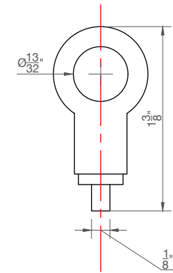
ELEVATION · OPTION C · GRIPPER RING SCALE · 1:1
