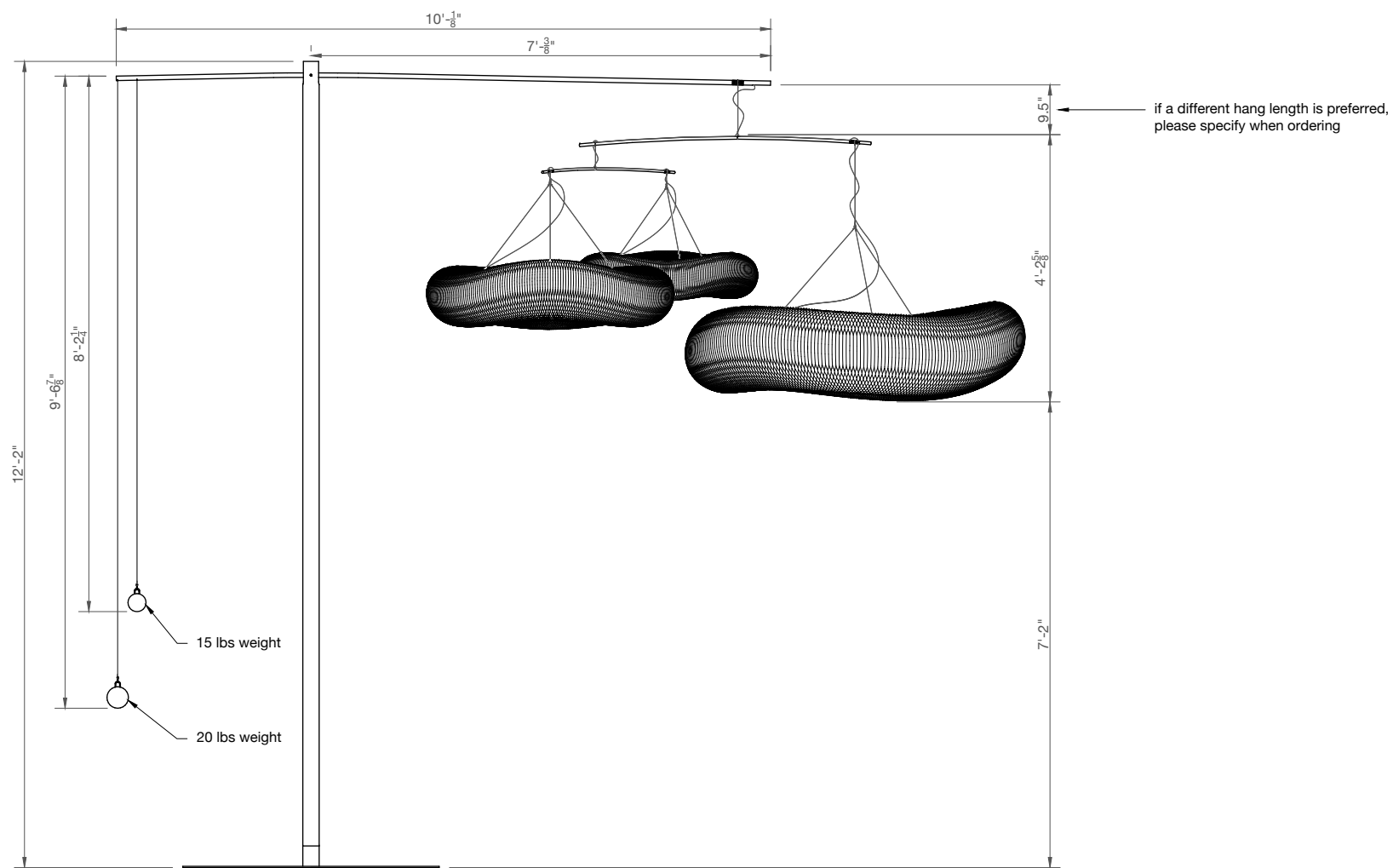
ELEVATION
