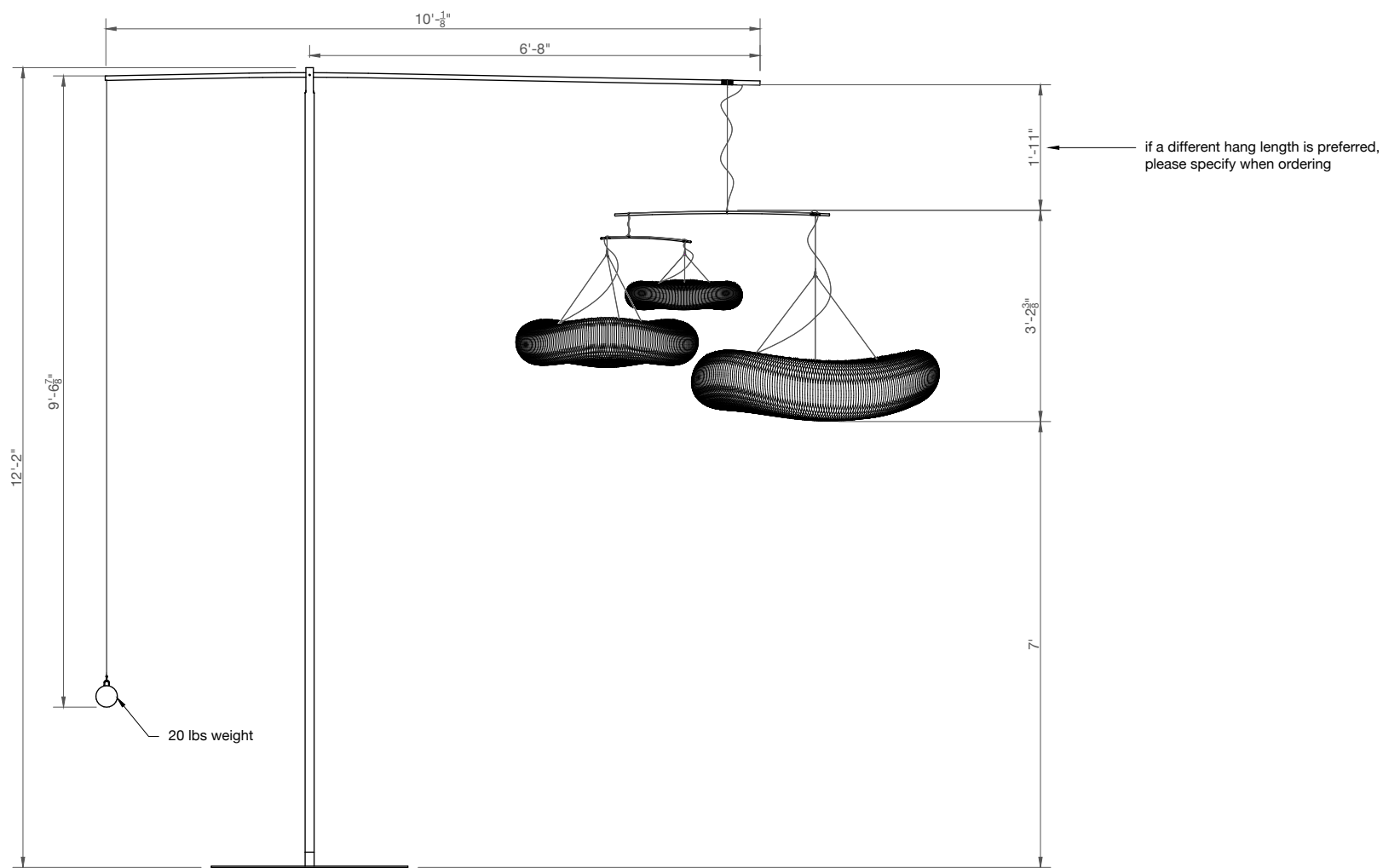
ELEVATION
