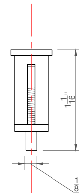
ELEVATION · OPTION B · SIDE EXIT GRIPPER SCALE · 1:1
