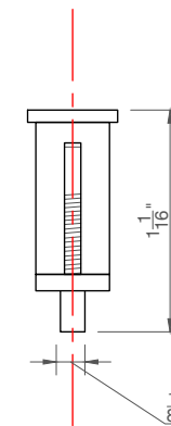
ELEVATION · OPTION B · SIDE EXIT GRIPPER SCALE · 1:1
