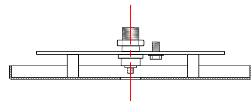
ELEVATION OPTION A · HANG KIT · CLOUD PENDANT
