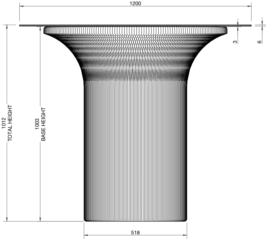
ELEVATION
