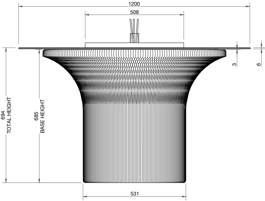
ELEVATION
