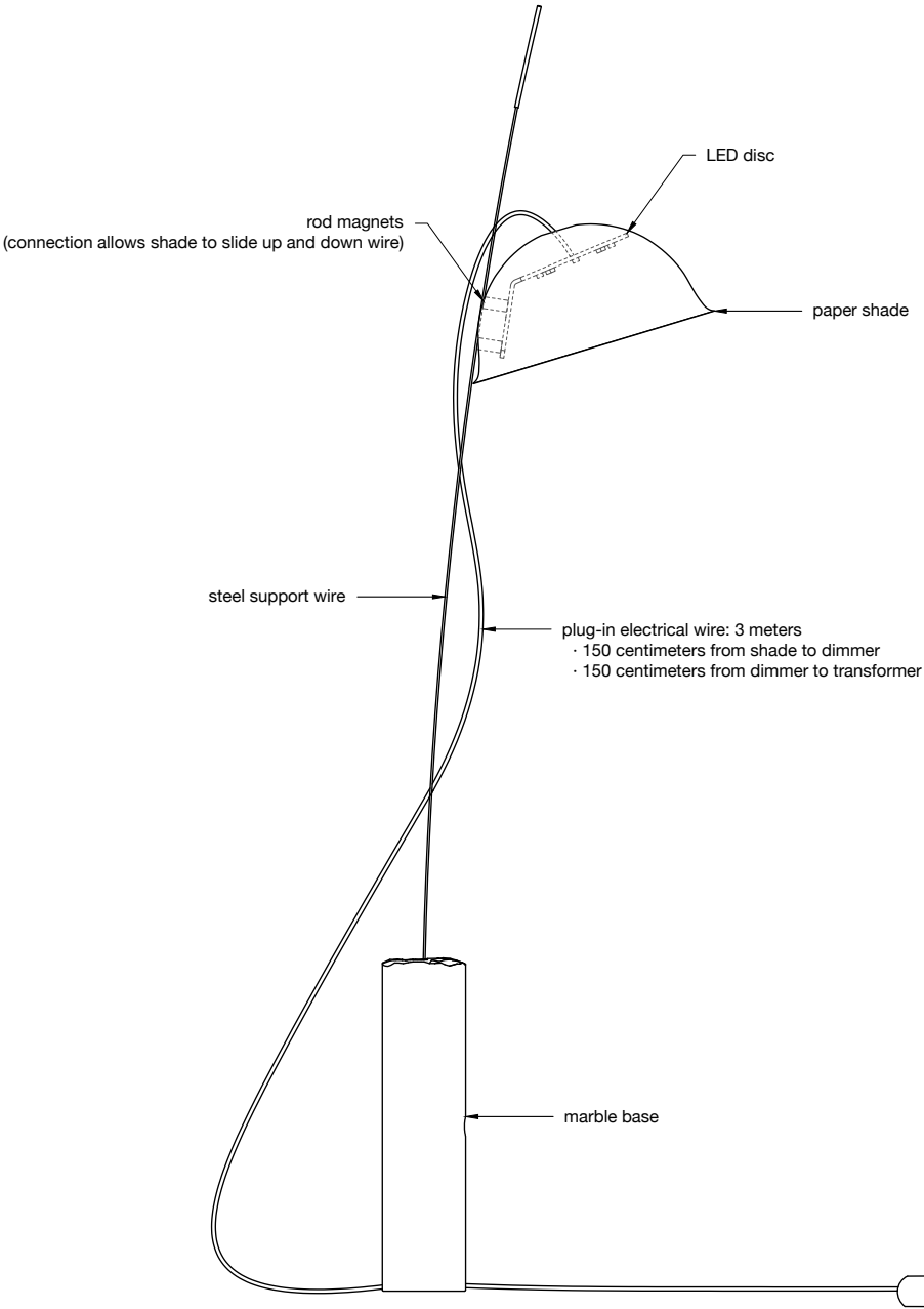
ELEVATION · SIDE
